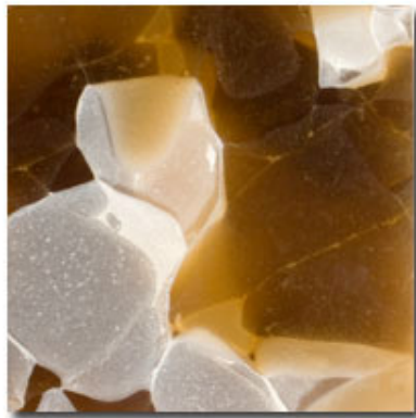
Zircon
