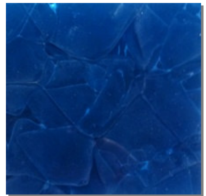
Tanzanite
